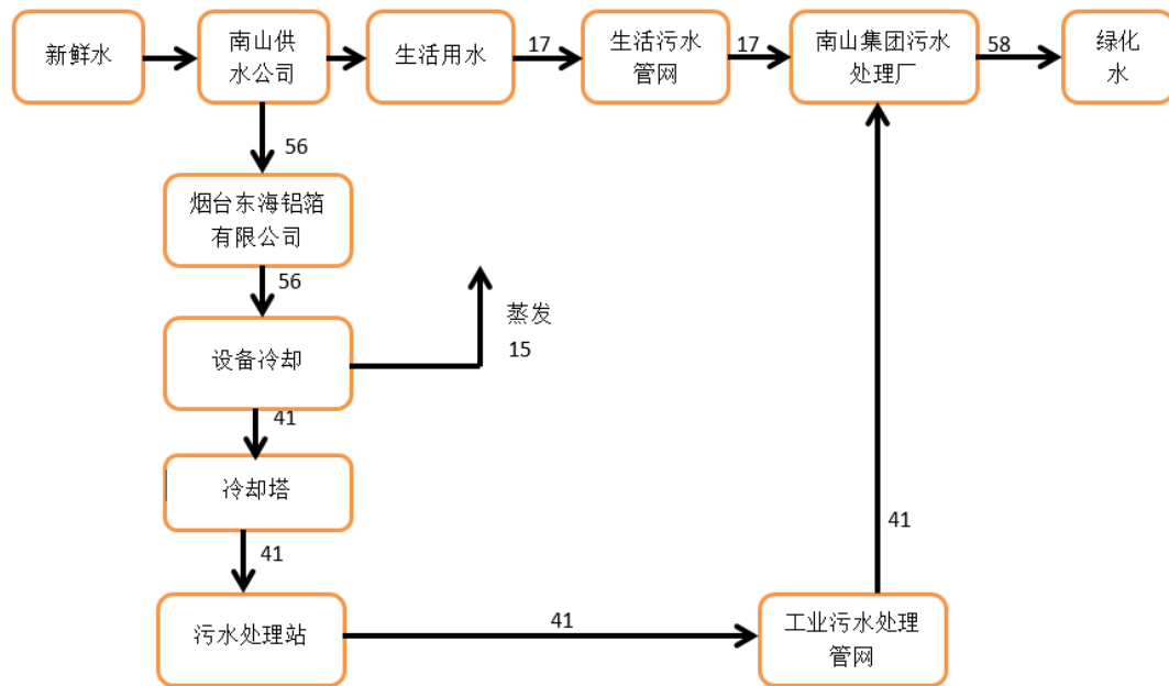
烟台东海铝箔有限公司水平衡图
